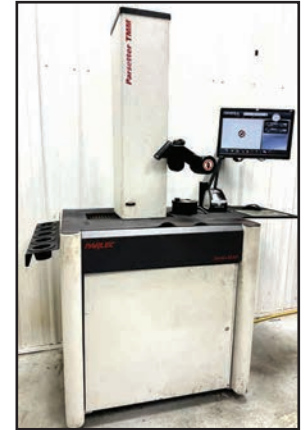
PARLEC PARSETTER TMM TOOL PRESETTER
